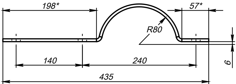
Поз.5 (Полухомут) развертка
