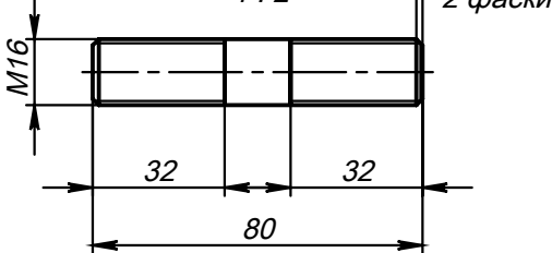
Поз.6 (Шпилька)
