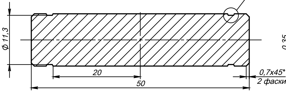
A-A (2:1)
