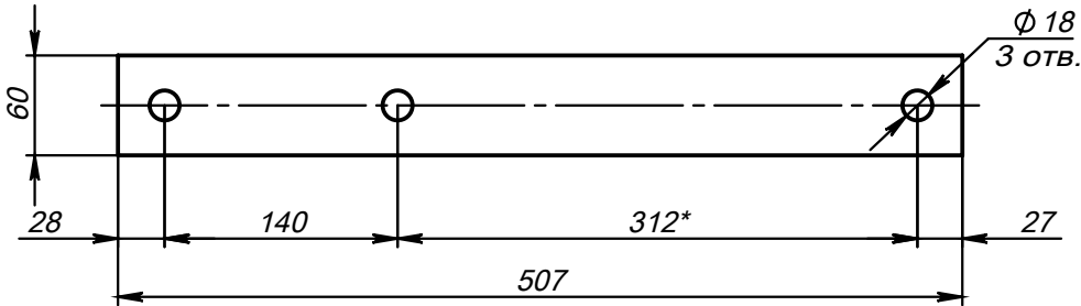
Поз.5 (Полухомут) развертка
